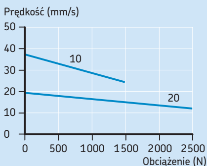
Prędkość w funkcji Obciążenia (siły)
